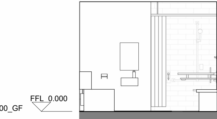
Elevation C 1 : 50
