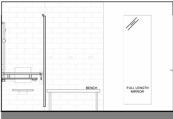
Elevation D 1 : 50
